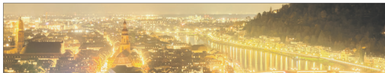
Licht aus! Künstliche Beleuchtung überstrahlt in der Stadt den Sternenhimmel.
